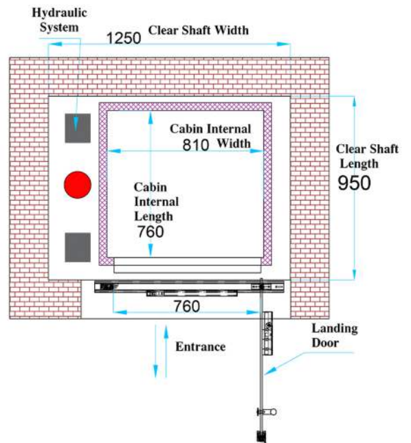
H250C Mini Elevator in Core
