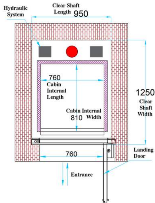
H250C Mini Elevator in Core
