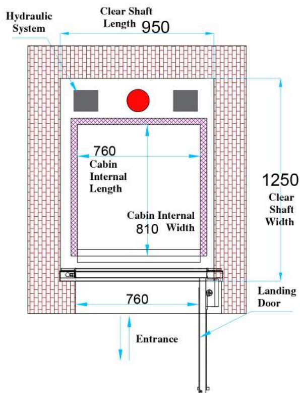
H250C Mini Elevator in Core
